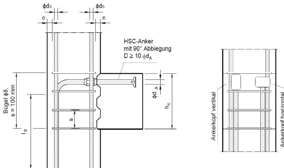
Abbildung 9: Bewehrungsführung von um 90^\circ nach unten abgebogenen HSC-Ankern in der Stütze, Beispiel
