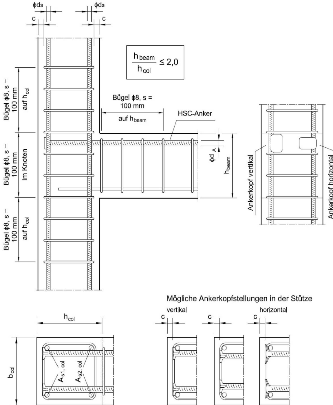
Abbildung 1: Bewehrungsführung, Beispiel
