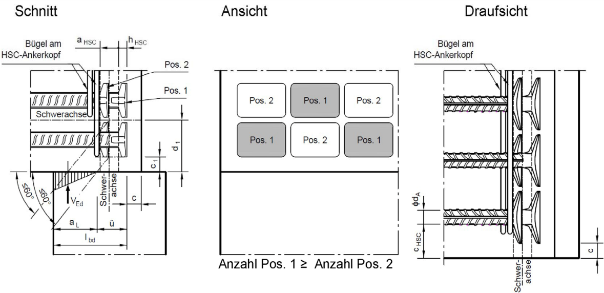
Abbildung 12: Anordnung zweilagig gestaffelter HSC-Anker mit dreiecksförmiger Lagerpressung, Beispiel
