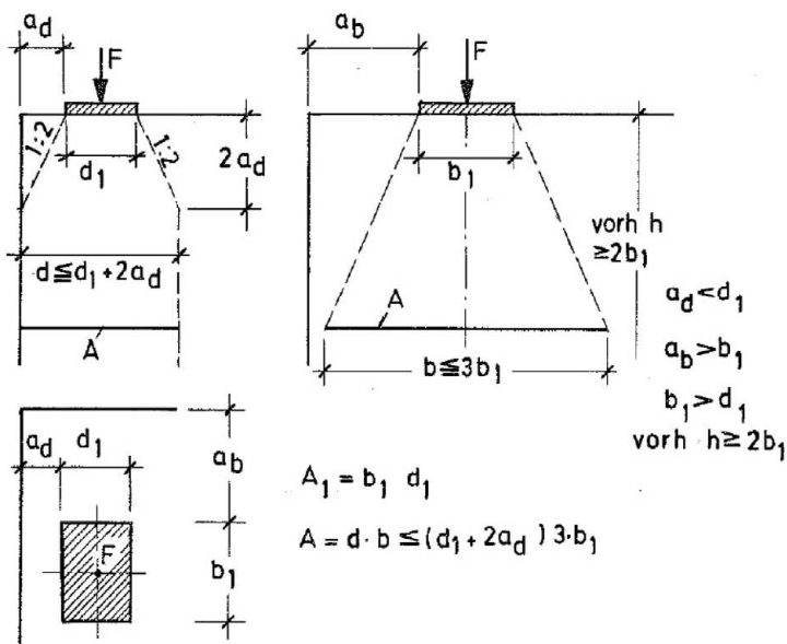
Abbildung 6: Bestimmung der rechnerischen Verteilungsfläche A_{c1} (= A) nach Leonhardt (Vorlesung über Massivbau – Teil 2: Sonderfälle der Bemessung im Stahlbetonbau)
