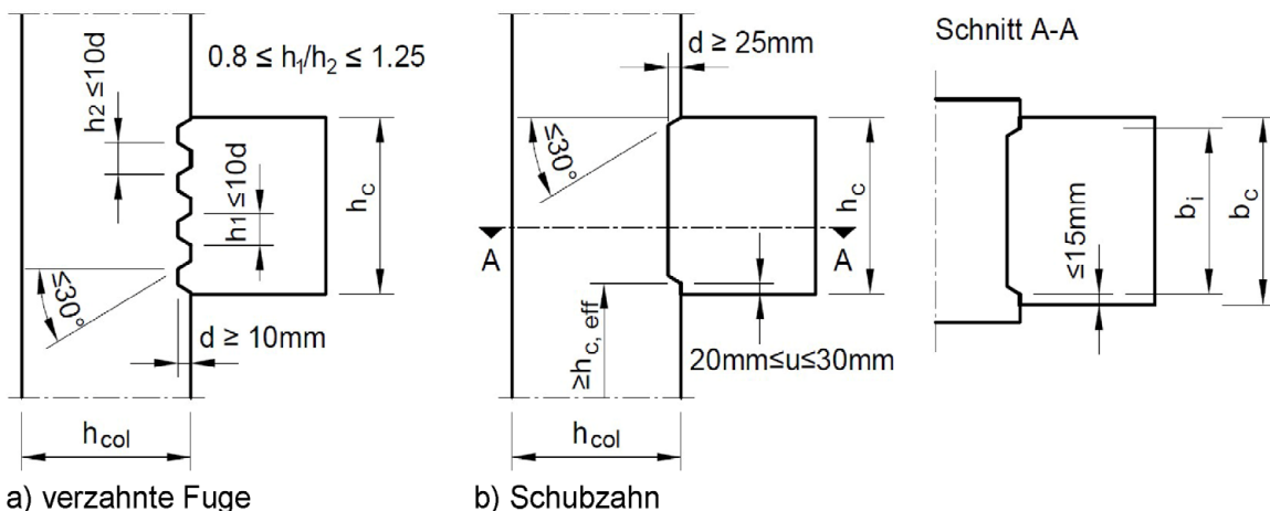
Abbildung 10: Ausbildung der Schubfuge
