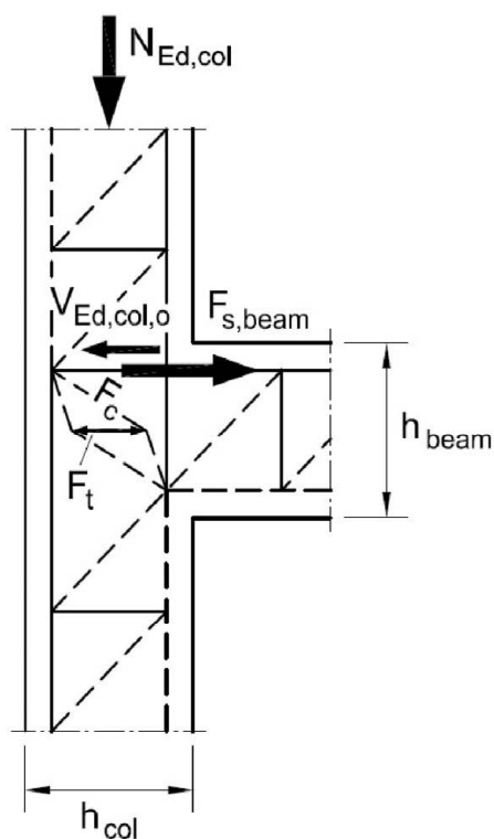
Abbildung 2: Stabwerkmodell
