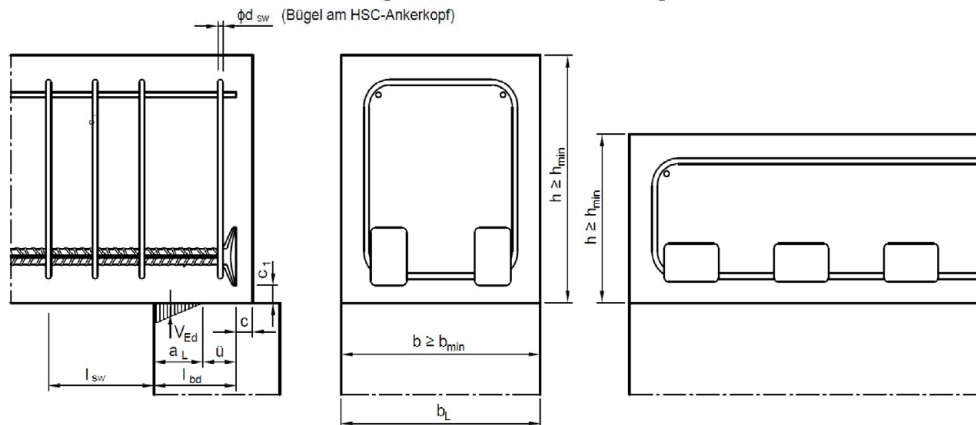
Abbildung 11: Anordnung der HSC-Anker mit dreiecksförmiger Lagerpressung, Beispiel
