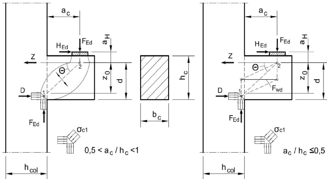
Abbildung 3: Stabwerkmodell nach DAfStb-Heft 600
