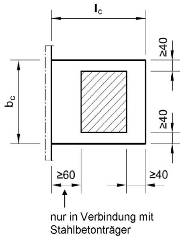
Abbildung 4: Anordnung einer Lasteinleitungsplatte, Empfehlung
