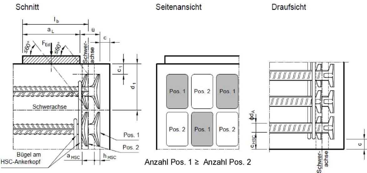
Abbildung 5: Anordnung der zweilagig gestaffelten HSC-Anker, Beispiel
