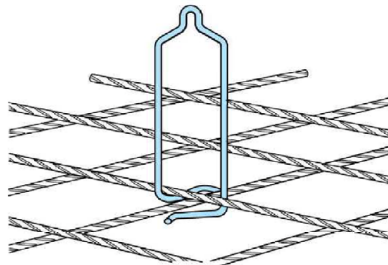
Bild 9: In senkrechte Lage schwenken.
