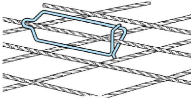
Bild 8: Einhängen wie dargestellt unter den oberen Bewehrungsstab.
