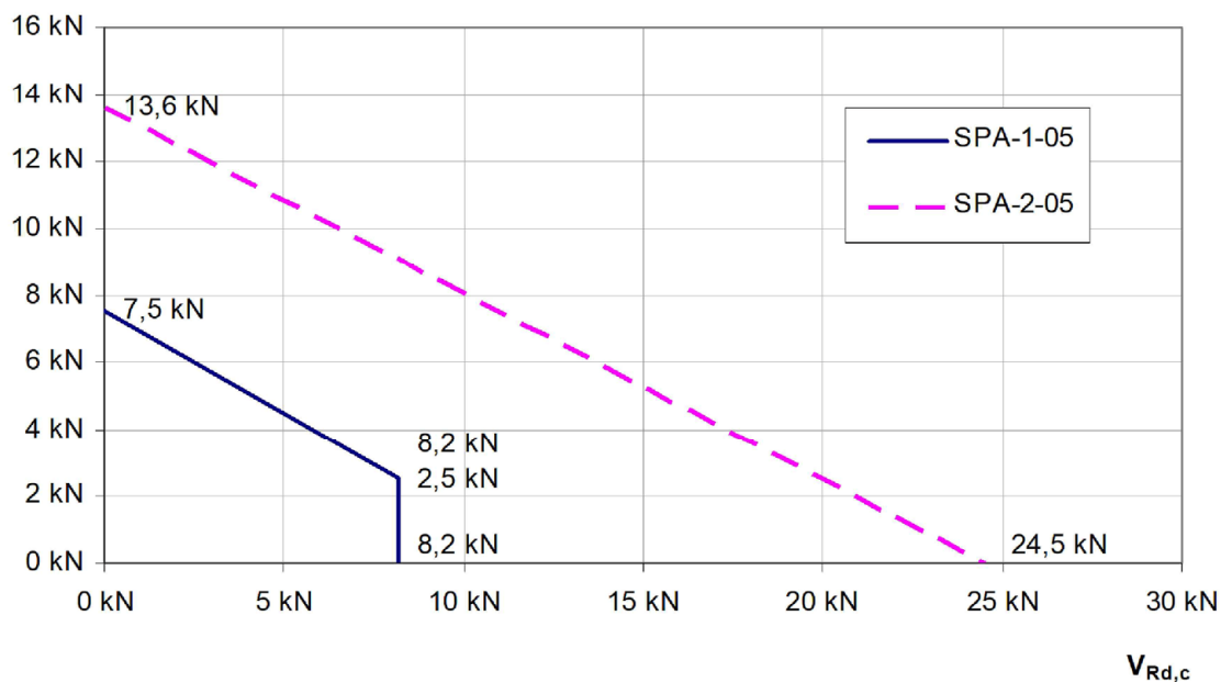
Diagr. 1: Betontragfähigkeitslinie SPA-05
