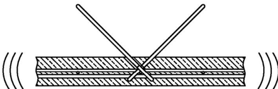
Bild 11: Verdichten der unteren Schicht. Einhalten der Ankerlängen im Beton gemäß Anlagen 4 und 6.
