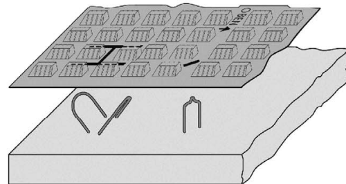
Bild 12: Vor dem Verlegen im Bereich der Anker Schlitze in die Distanzhalterplatte schneiden.
