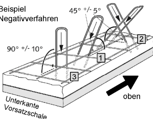
Bild 17: Spätestens 60 min nach Zugabe des Anmachwassers Verbundnadel durch die Wärmedämmung bis an den Schalungsboden drücken und gegebenenfalls auf das erforderliche Einbindemaß herausziehen.
