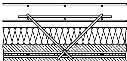
Bild 19: Obere Schicht bewehren, SPA-1 /-2 entsprechend Anlage 4 einflechten (siehe auch Bilder 1 - 4.) Einhalten der Ankerlänge im Beton gemäß Anlagen 4, 5 und 6.
