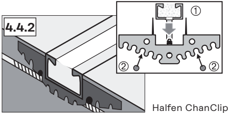
Halfen ChanClip
