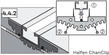
Halfen ChanClip
